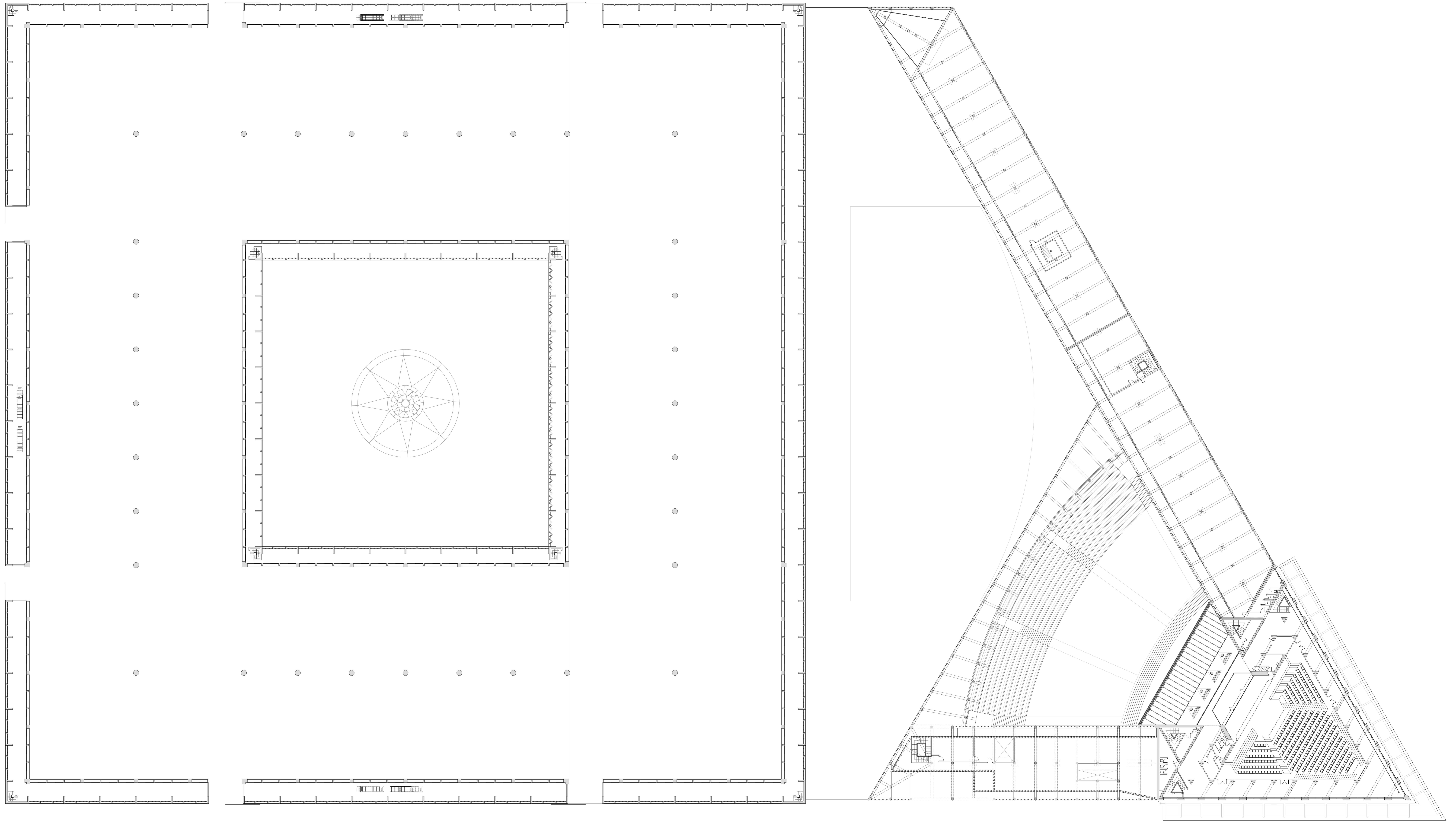
PLANTA PRIMERA COTA +3.00
